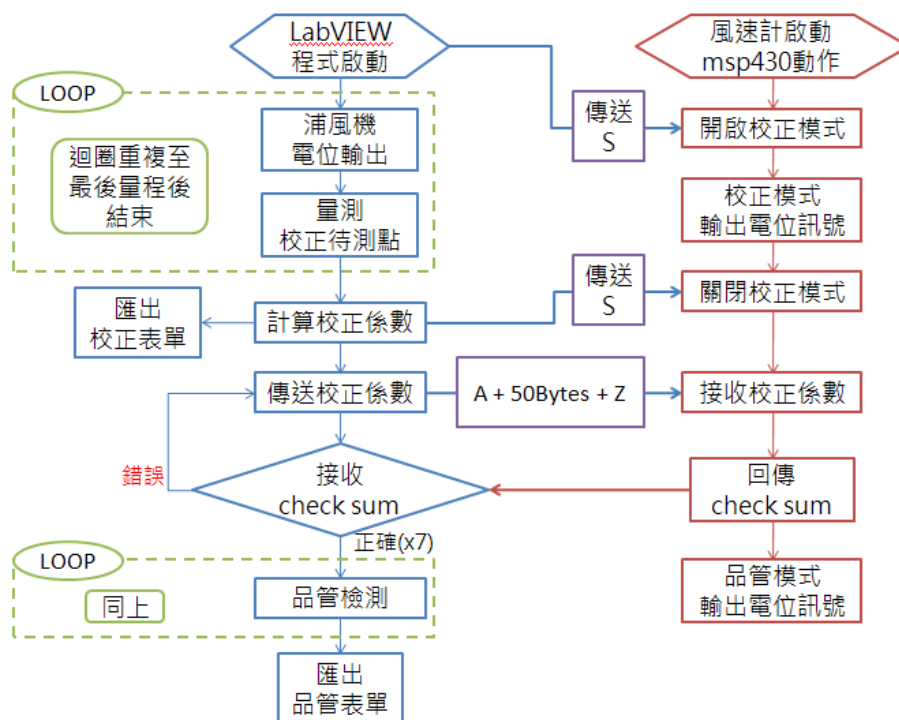
圖 7 通訊程式架構圖
