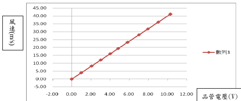
圖 15 線性校正後之電壓對應風速曲線(40m/s)
