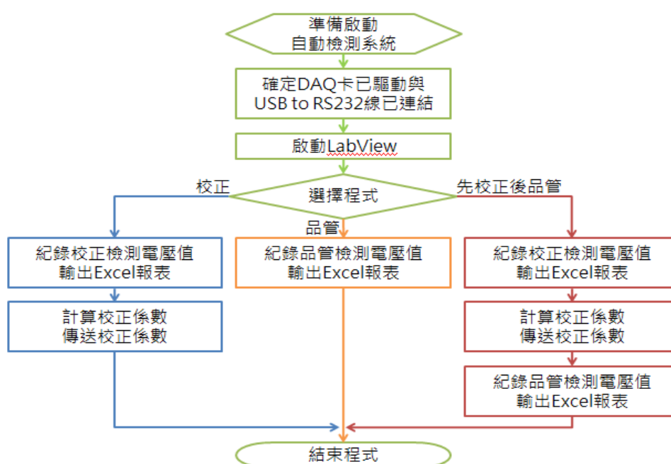
圖 10 熱線式風速計線性校正與品管程式流程圖
